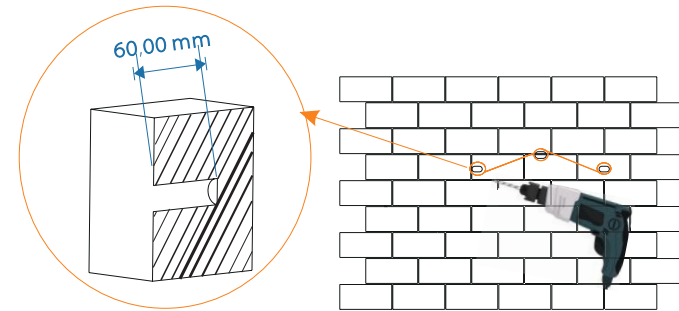
Taladro Ø10 mm (Profundidad: 60 mm)
